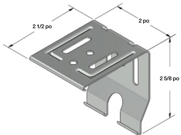
Supports requis par largeur
