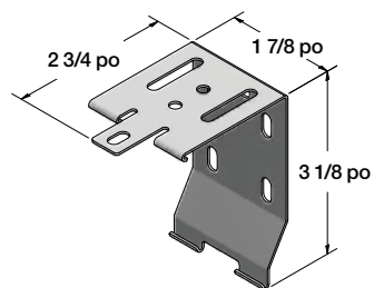
Supports requis par largeur
